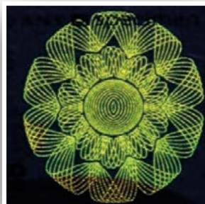
UV 313 nm
